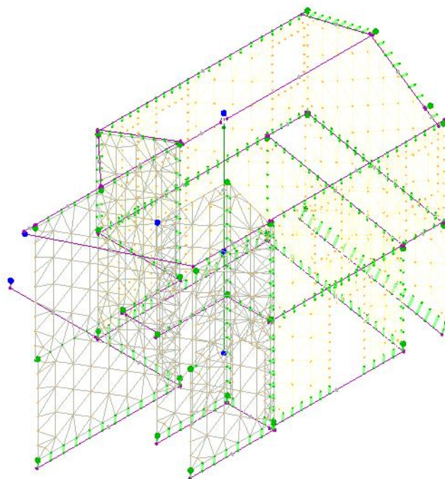
Vista Posteriore
